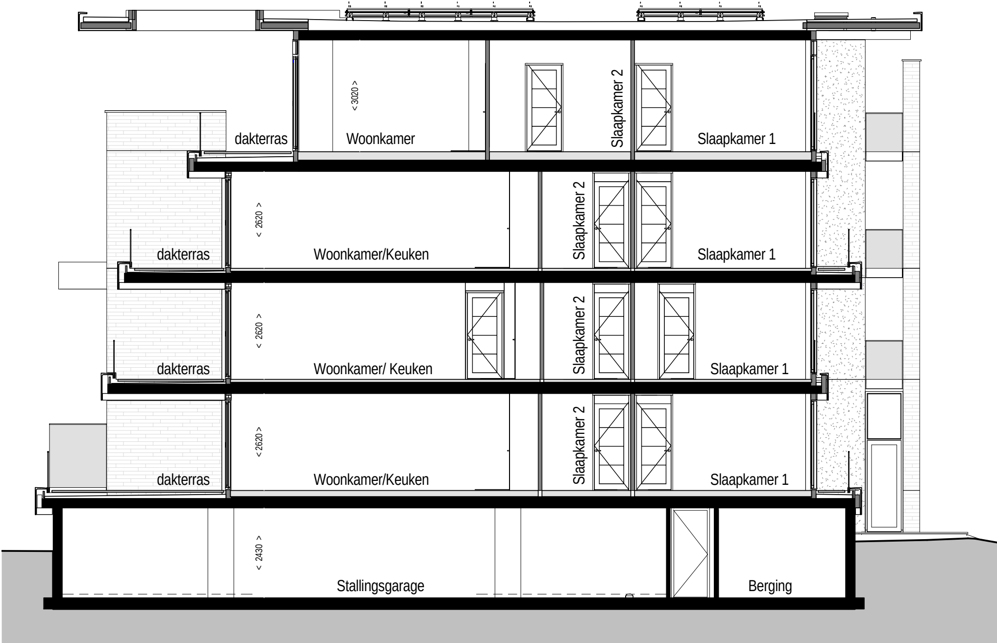
DOORSNEDE A-A
