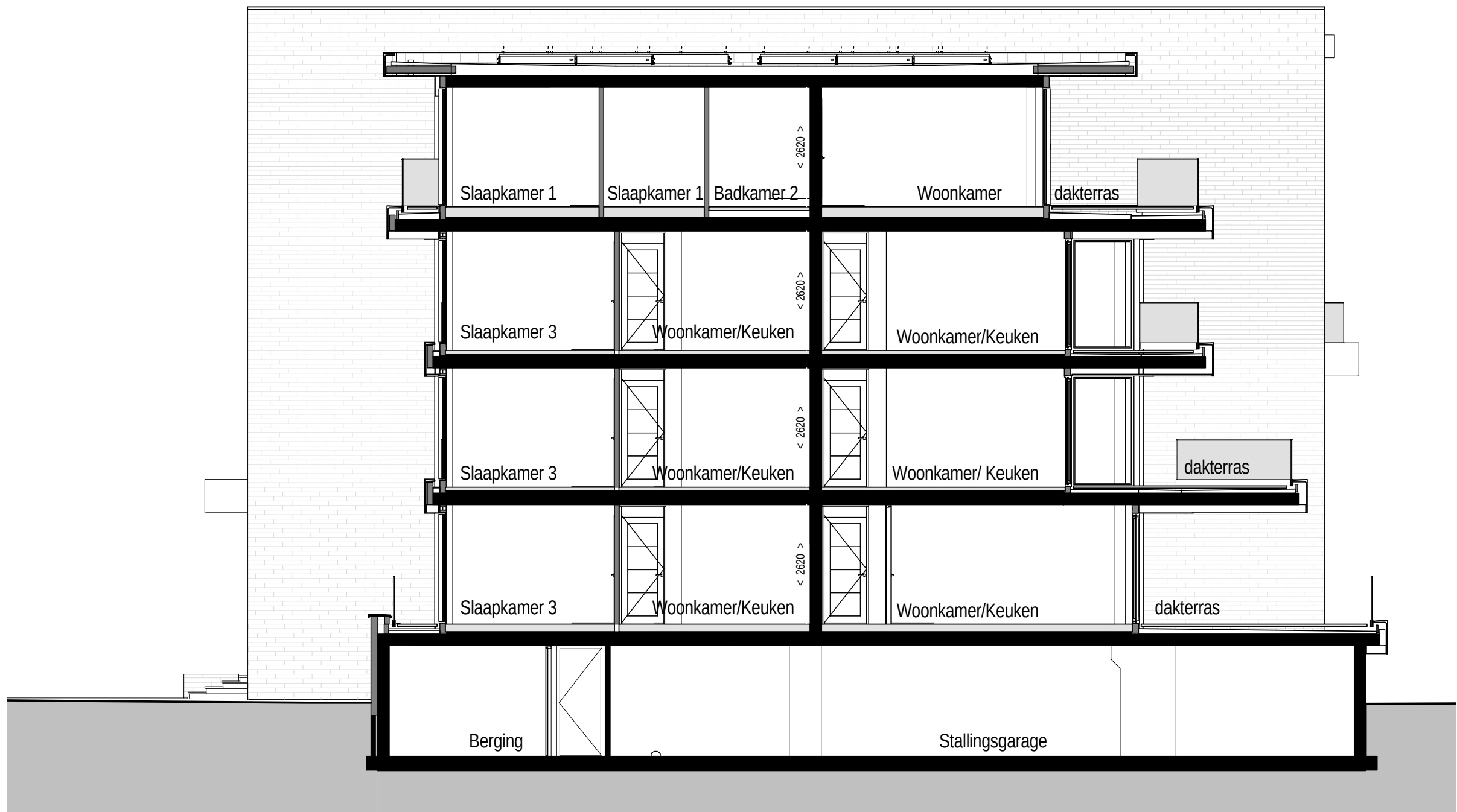
DOORSNEDE B-B
