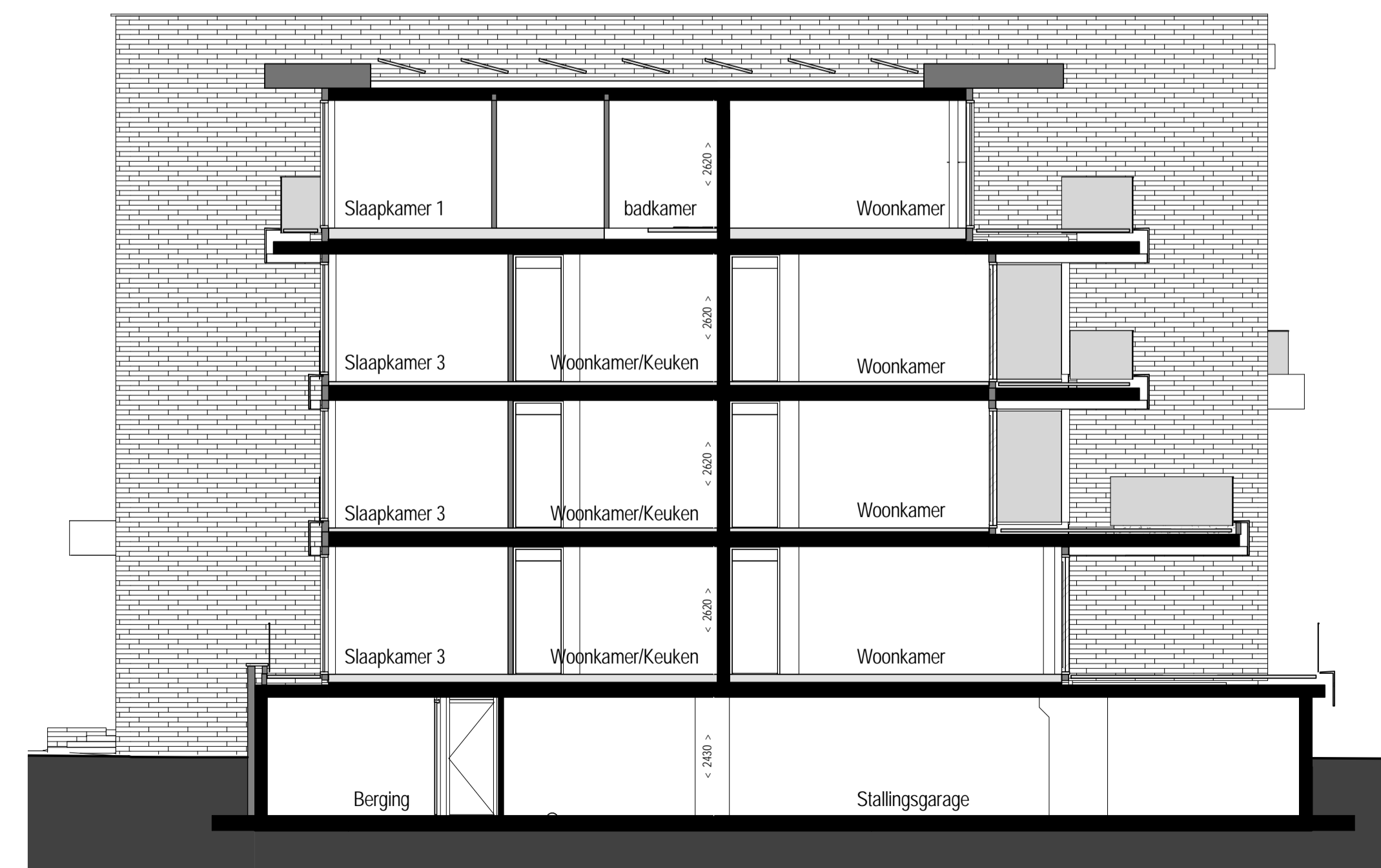
DOORSNEDE B-B
