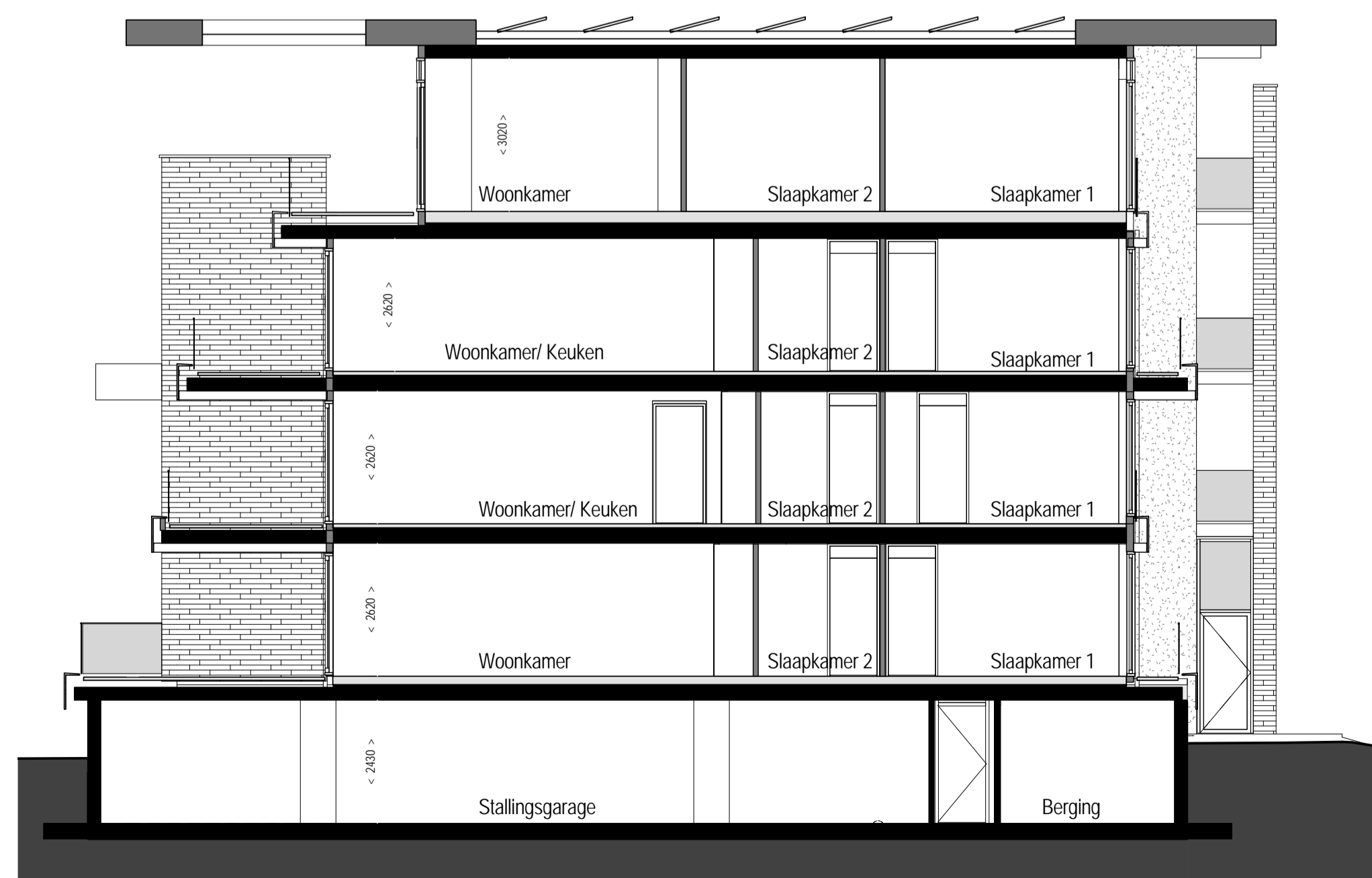
DOORSNEDE A-A
